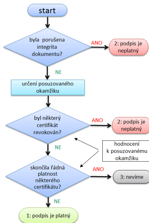
Obrázek 3-2: Vývojový diagram - postup ověřování platnosti elektronického podpisu
