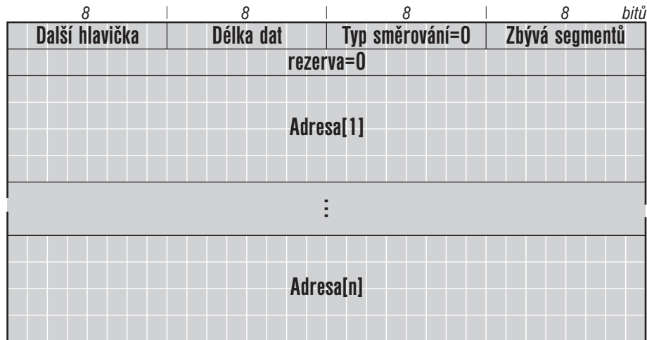
Obrázek 2.7: Rozšiřující hlavička Směrování typu 0
