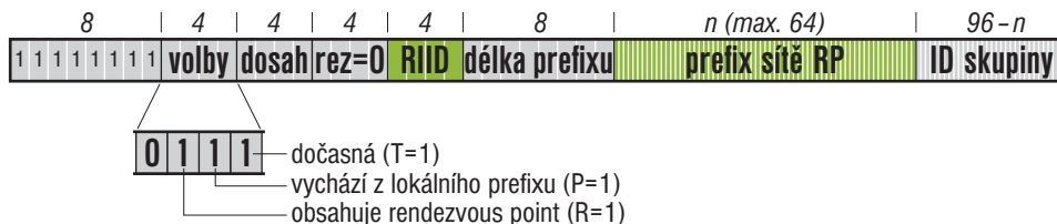
Obrázek 3.12: Skupinová adresa obsahující RP
