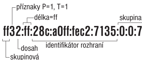
Obrázek 3.11: Příklad adresy založené na identifikátoru rozhraní
