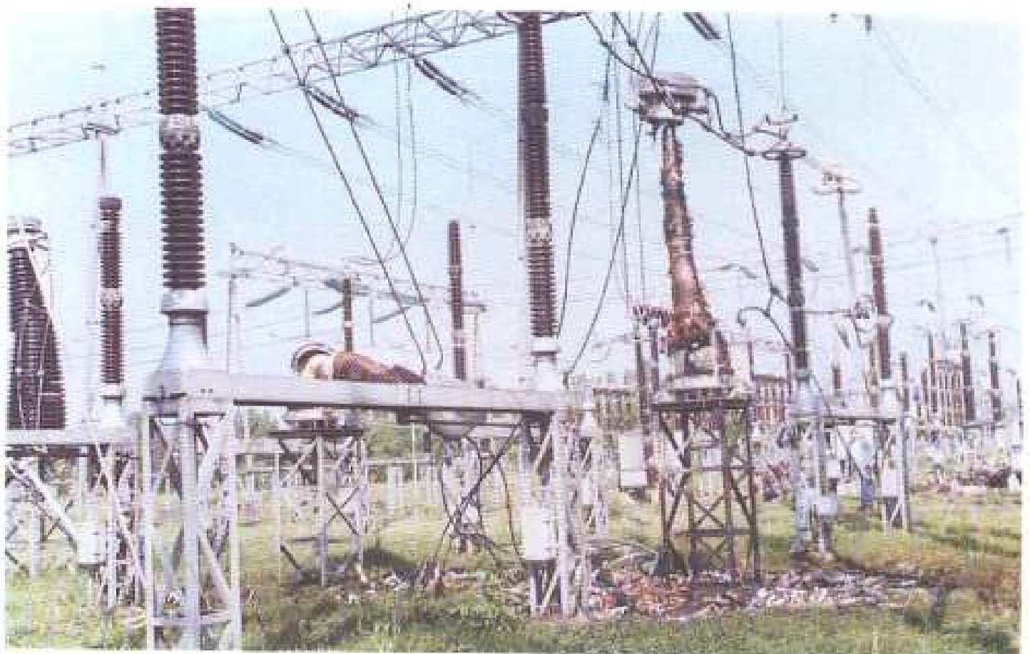
Слика 53 Оштећења на главном систему Сабирница трафо-станице „Београд 8” у Лештанима
