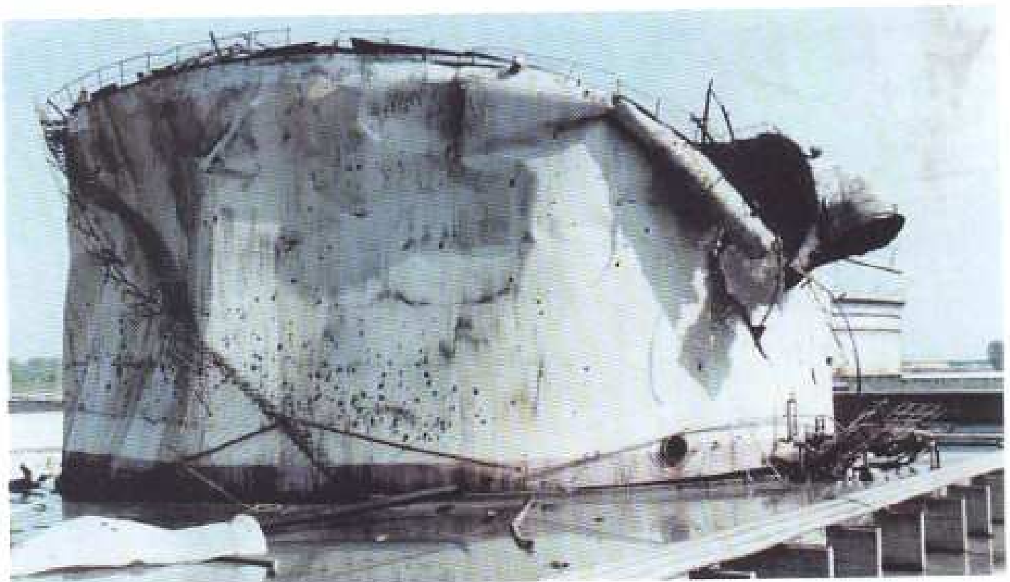
Слика 2 Уништени резервоар Р-24
