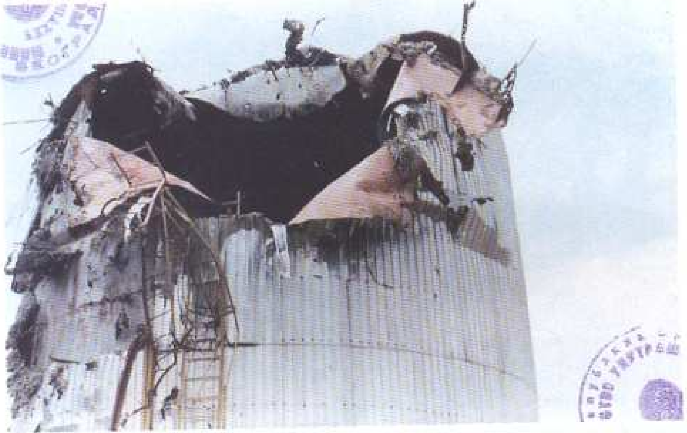
Слика 14 Разорени резервоар у складишту горива „Југопетрола“ у Бору у дане 15. и 17. 05. 1999. године
