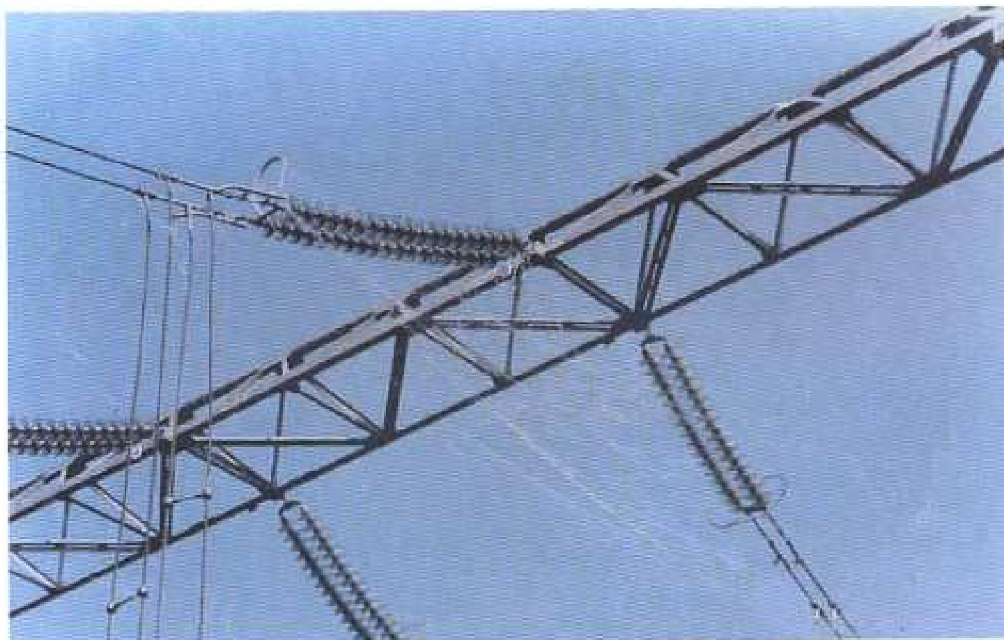
Слика 4 Ближи изглед карбонских влакана који су направили кратак спој на високонапонским кабловима
