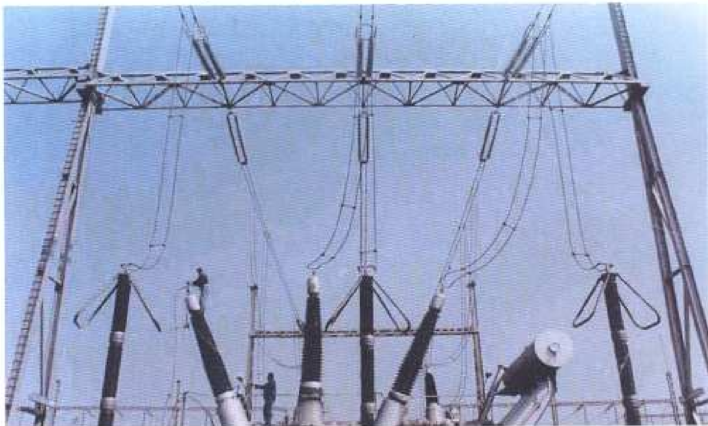
Слика 3 Разводно постројење са трансформатором Термоелектране „Никола Тесла“ у Обреновцу на које су бачене касетне бомбе са карбонским влакнима који су изазвали кратке спојеве и испадање система дана 02. 05. 1999. године
