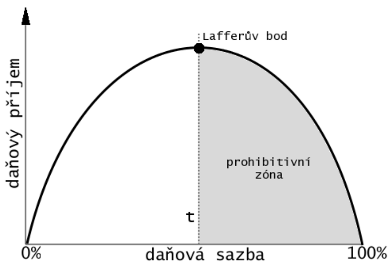
Lafferova křivka
