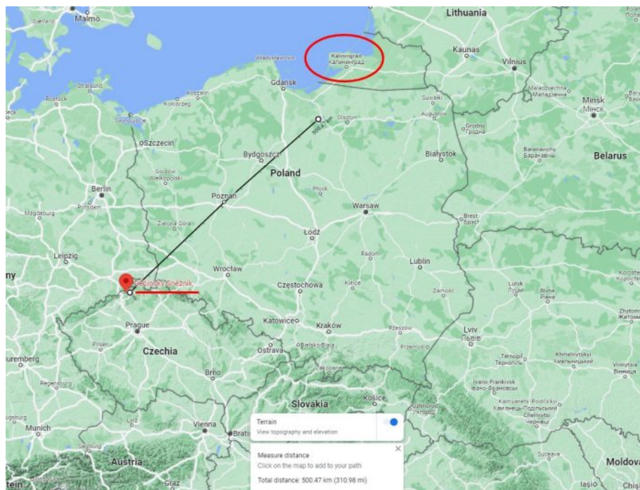
Jmenovitý dosah radaru VERA-NG ve směru na Kaliningradskou oblast Ruské federace
