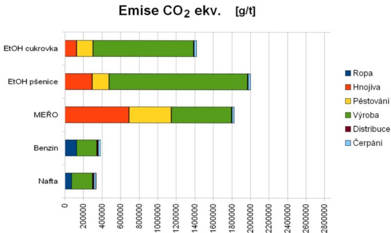
Emise CO 2 podle druhu paliva, zdroj: Centrum dopravního výzkum, graf: Kverulant.org
