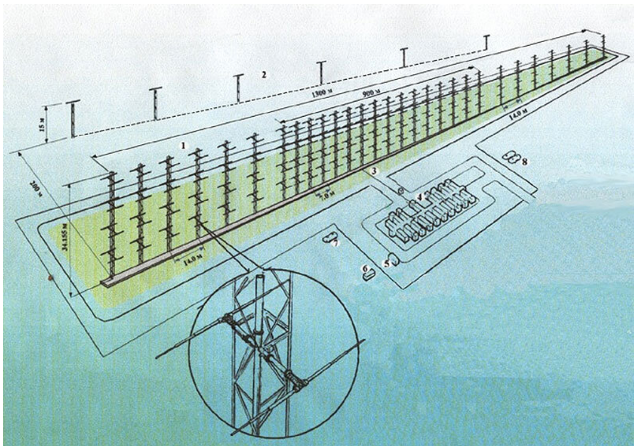
Ruský radar Container, technický náčrt. Délka 1300m, výška 34 metrů.
