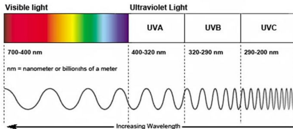
Vlnové délky spojitého světelného spektra
